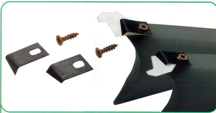
PIASTRINE BLOCCA RASCHIETTO COMPLETE DI VITI SCRAPER HOLDER PLATE COMPLETE WITH SCREWS PLACA FIJADORA DEL RASCADOR CON TORNILLO
