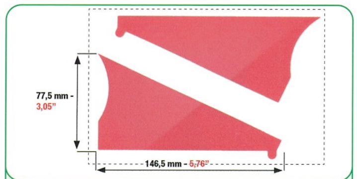
ADESIVI PER SPALLE DI BLOCCAGGIO COPRICALAMAIO PER: ADHESIVES FOR INK DUCT END BLOCKS FOR: ADHESIVOS PARA RESPALDO DE BLOQUEO DEL CUBRETINTERO PARA:
