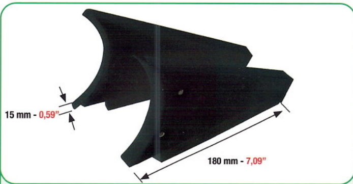
SPALLE DI BLOCCAGGIO COPRICALAMAIO PER: INK DUCT END BLOCKS FOR: RESPALDO DE BLOQUEO DEL CUBRETINTERO PARA:
