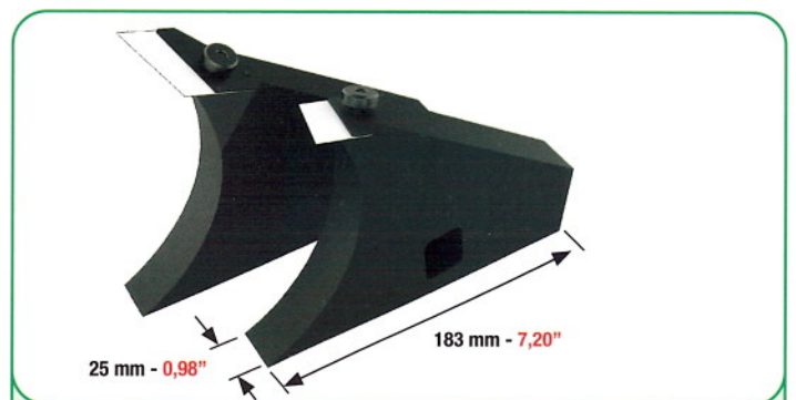
SPALLE DI BLOCCAGGIO COPRICALAMAIO COMPLETE PER: COMPLETE INK DUCT END BLOCKS FOR: RESPALDO COMPLETO DE BLOQUEO DEL CUBRETINTERO PARA:
