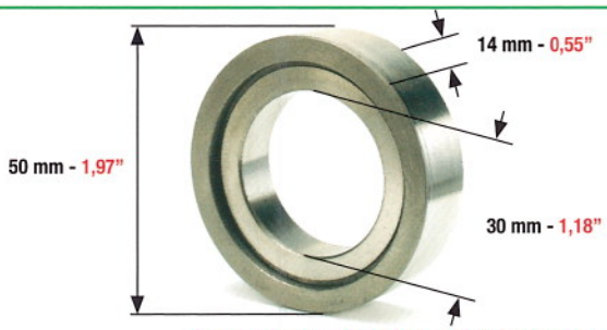
PLATINA PICCOLA 26x38 E PLATINA GRANDE 32x46 FOR PLATEN "T" 26x38 AND "GT" 32x46 PARA PLATINA MINERVA "T" 26x38 - PLATINA MINERVA "GT" 32x46
