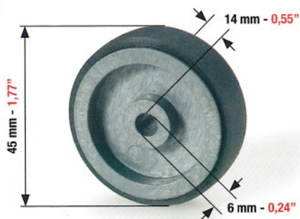
RUOTA DI TRASPORTO IN PLASTICA E GOMMA PER: FEEDER WHEEL IN PLASTIC AND RUBBER FOR: RUEDA DE TRANSPORTE DE PLÁSTICO Y GOMA PARA:
